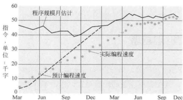
图 8-3 ESS 预计和实际的编程程度
