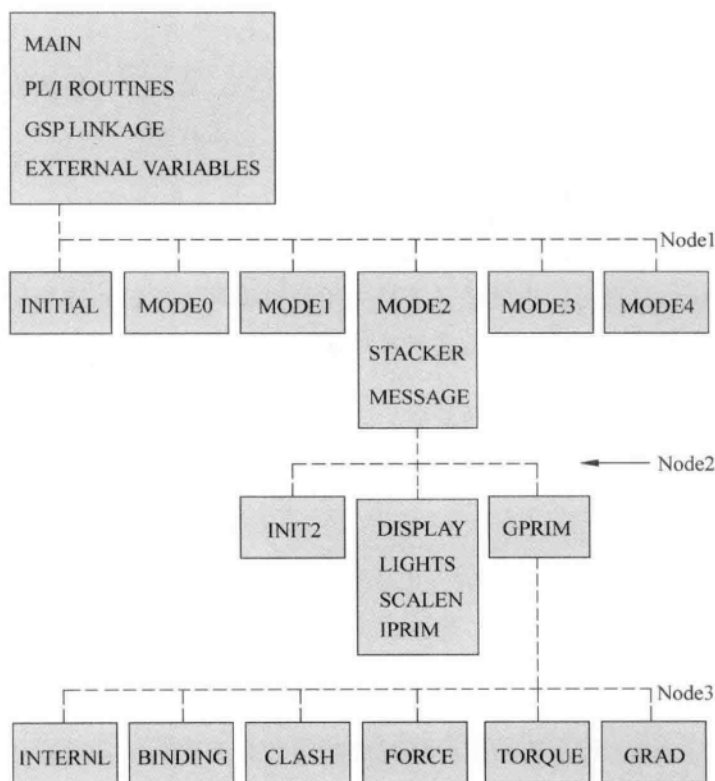
图 15-1 程序结构图(Courtesy of W.V. Wright)
