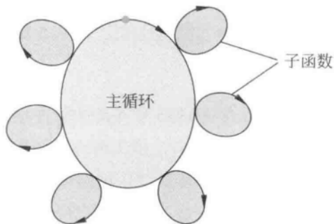
图 19-2 实时系统的基本轮询回路
